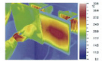
▲左が「サンバリア」を貼ったガラス。「サンバリア」を貼っていないガラスが30℃前後まで温度が上がっているにもかかわらず、「サンバリア」を貼ったガラスは18℃前後を保ったままの状態です。
